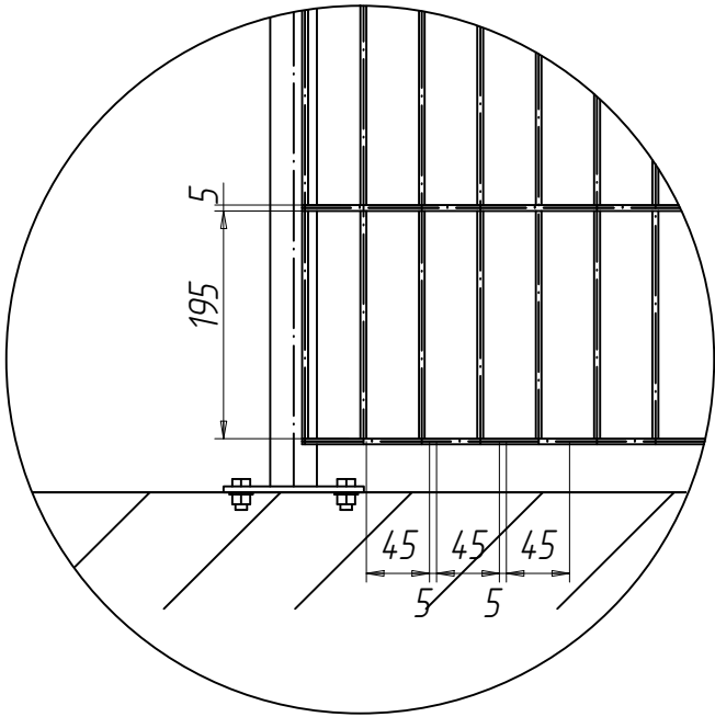
Узел - Б
