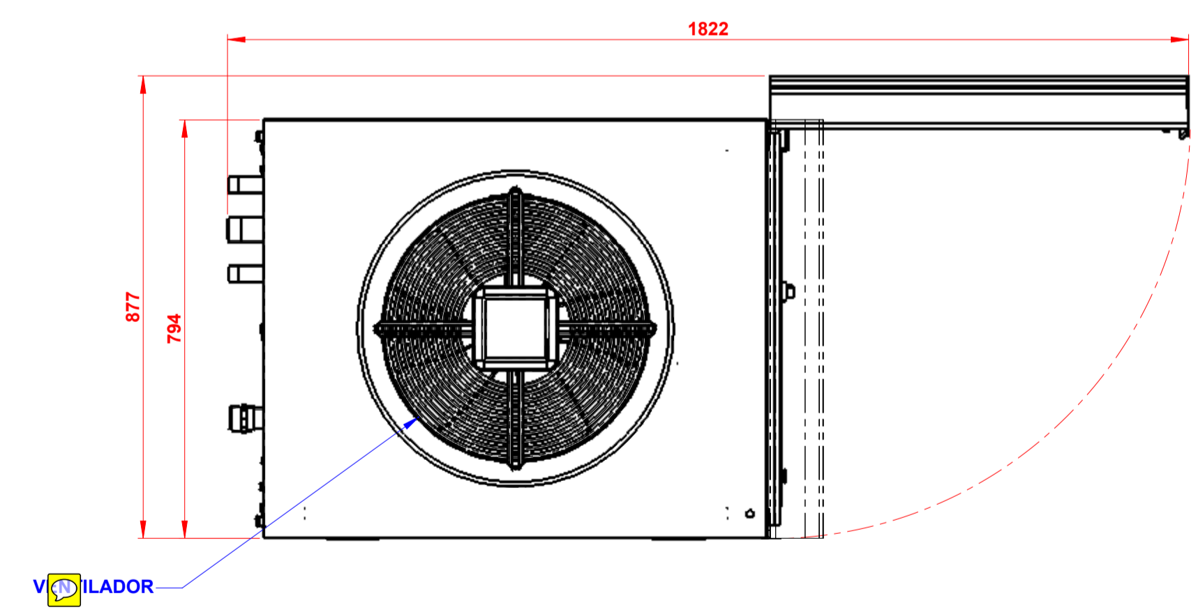
VISTA SUPERIOR
