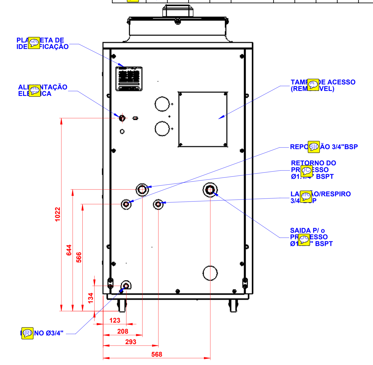
VISTA TRASEIRA
