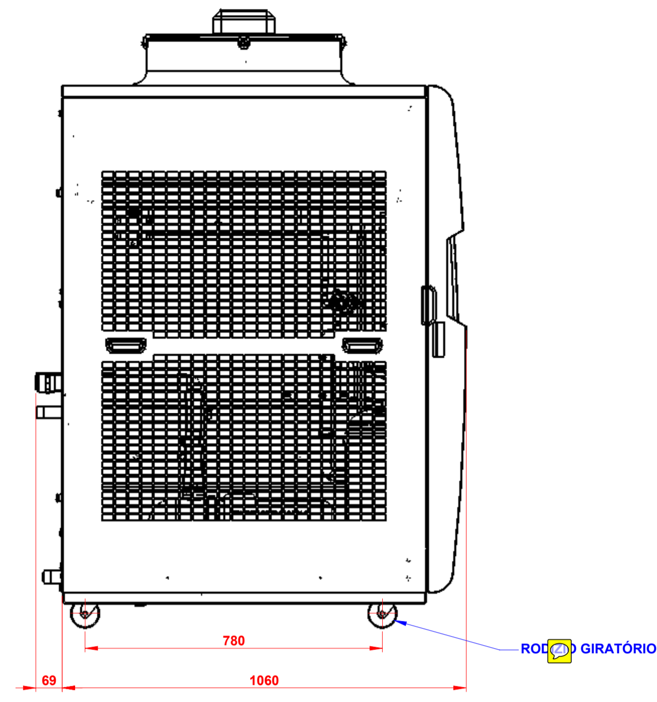
VISTA LATERAL
