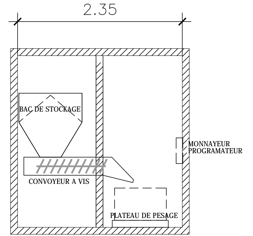
VUE LATERALE
