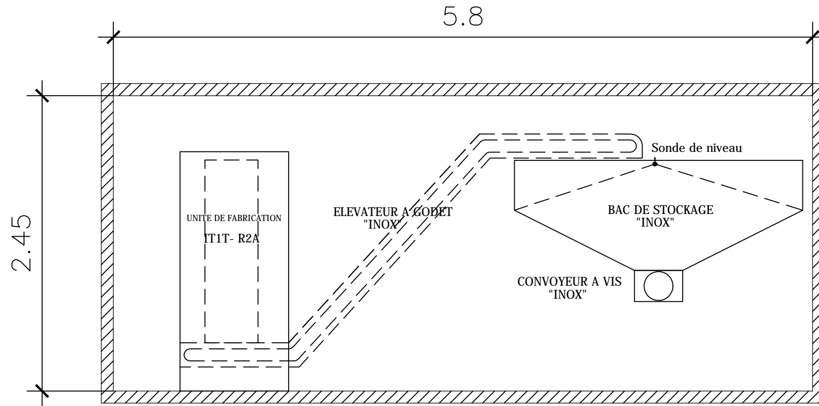
VUE TRANSVERSALE
