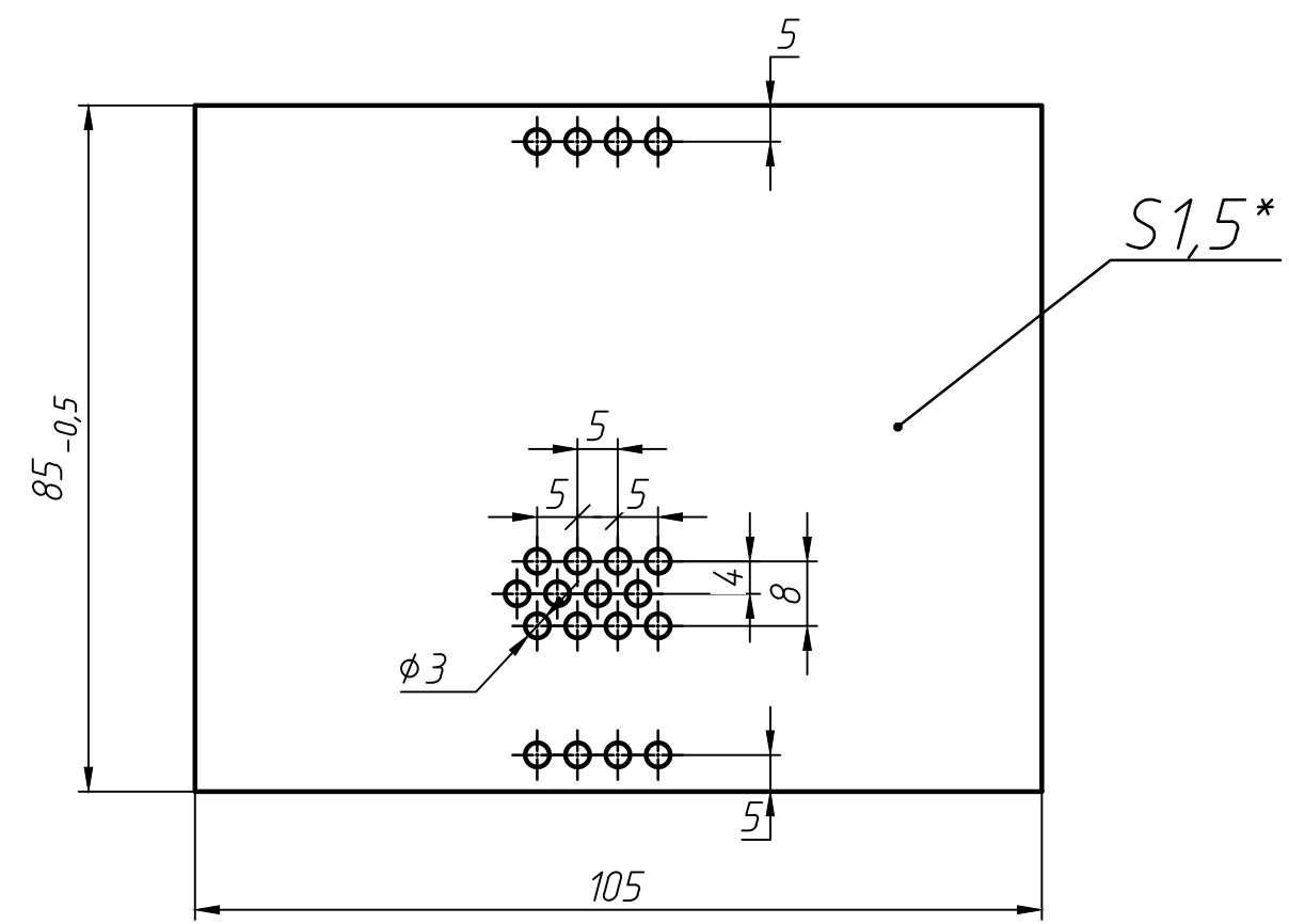
Развертка (1:1)
